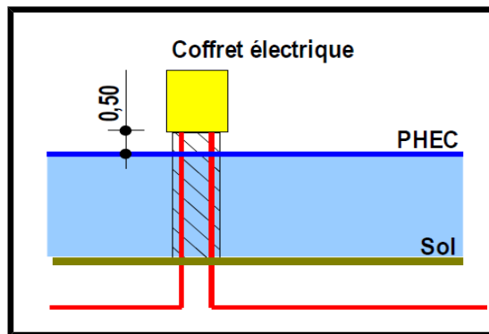
Illustration branchement des habitations
