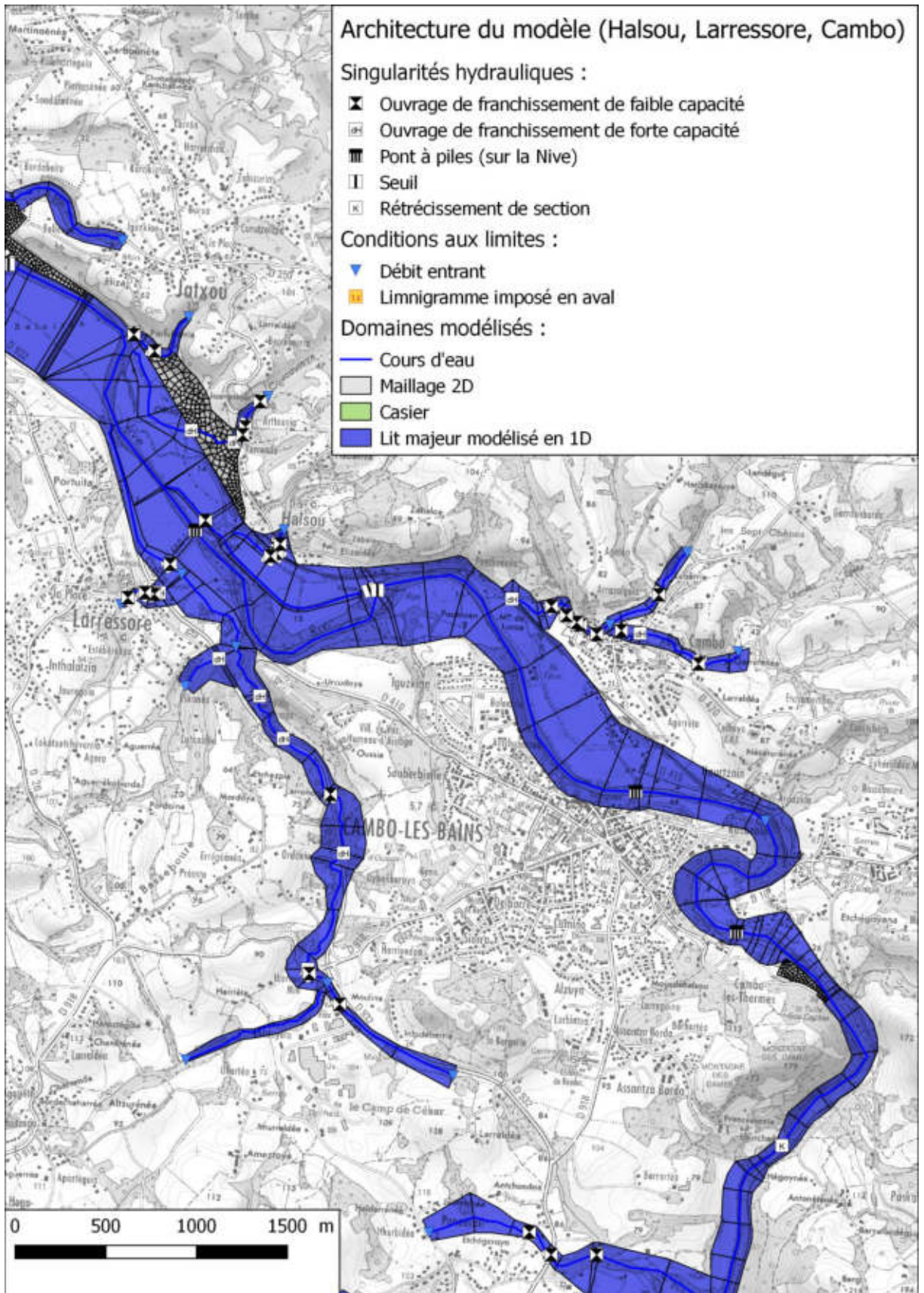
Figure 9 : Architecture du modèle au droit de Cambo-les-Bains
