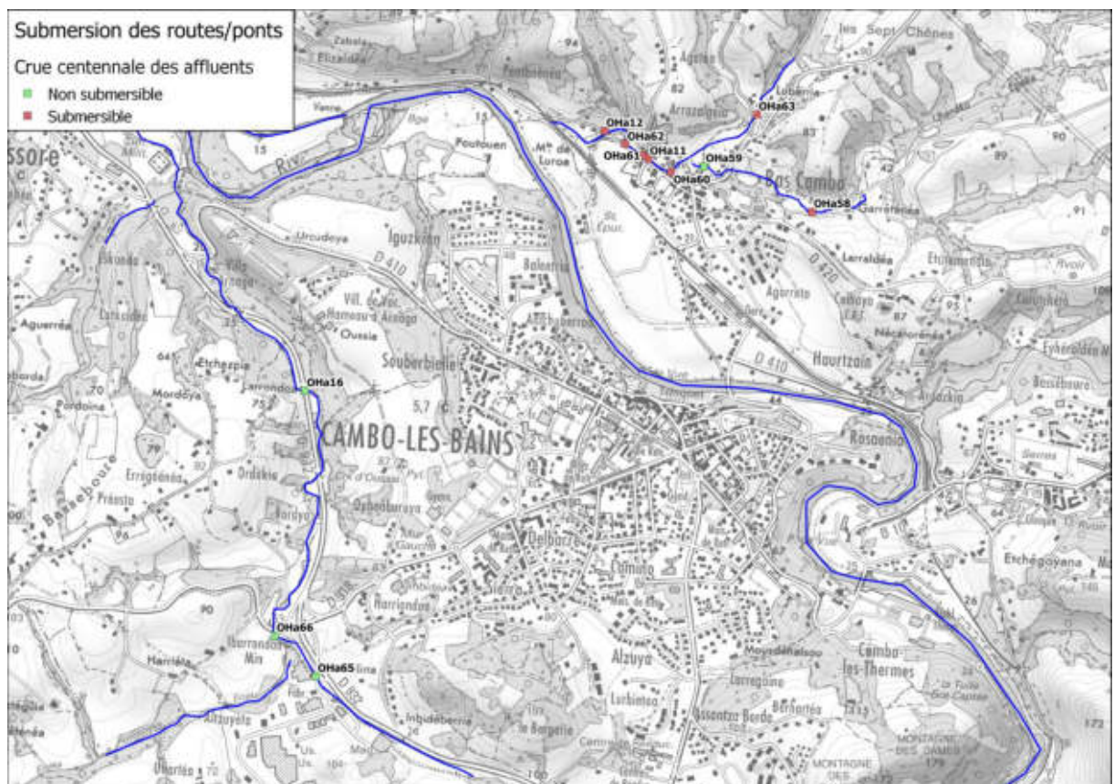
Figure 13 : Submersion des routes/pont au cours de la crue centennale des affluents – Cambo-les-Bains,
