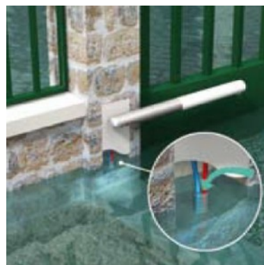
Passage possible de l'eau par les entrées de gaines
